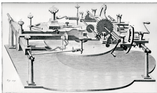
Macchina di Hulett dall'Encyclopédie ou Dictionnaire raisonné des sciences, des arts et des métiers
